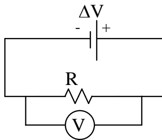
Figure 4.3.1. Méthode de branchement d'un voltmètre
