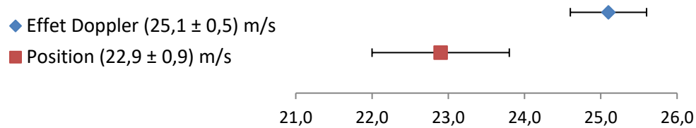
Figure 4.4.1. Diagramme de comparaison des mesures de vitesse - chevauchement
