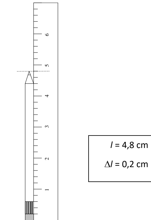
Figure 3.5.2: Incertitude absolue pour l'utilisation d'une règle
