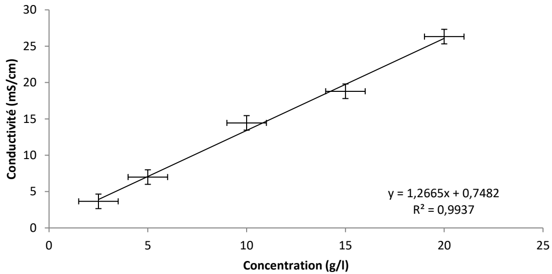
Figure 4.4.1. Conductivité de la solution en fonction de sa concentration en sel.
